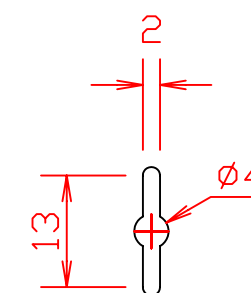
A部穴詳細図(2箇所)
