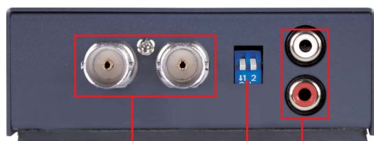
HD/SD-SDI 入出力コネクタ (アクティブスルーアウト)
