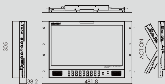
■TLM-170GR 7Uサイズ19インチラックマウント型
