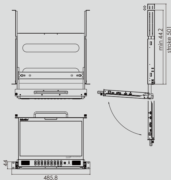
■TLM-170GM 1Uサイズ引出式19インチラックマウント型
