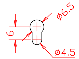
A部詳細図
