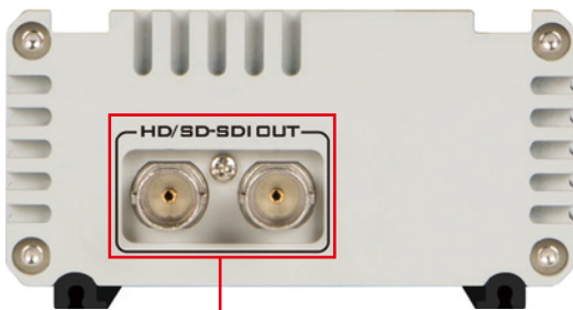
HD/SD-SDI 出カコネクタ
