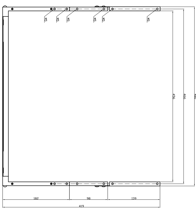
3U用付属金具取付
