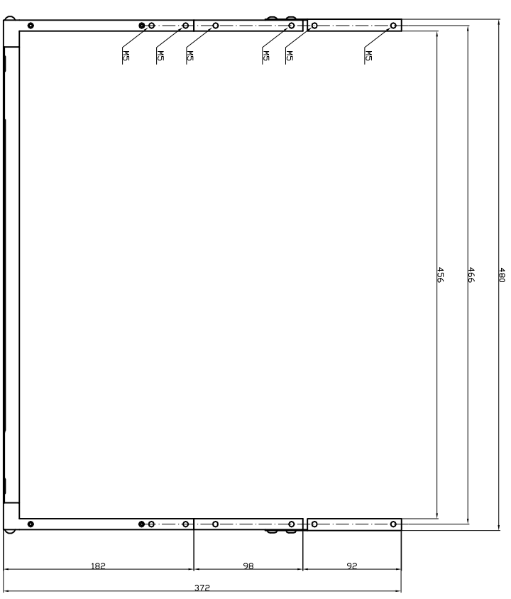
2U用付属金具取付
